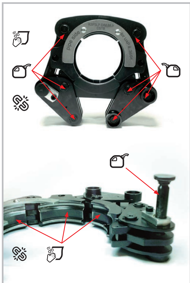
Fig. 19 – Klaukeutrustning
